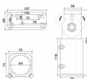
Adaptateur orientable pour extrémité de poteau
