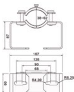
Adaptateur pour poteau
